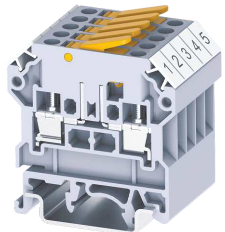
CKT4UH Terminals
