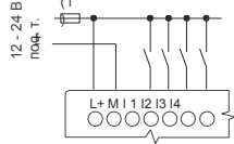
[Дискретный ввод - питание (пер. т.)]
