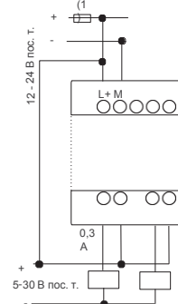
[Транзисторные выводы (ррр)]
