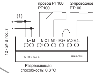
[соединение Pt100 (-50 ... +300 °C)]
