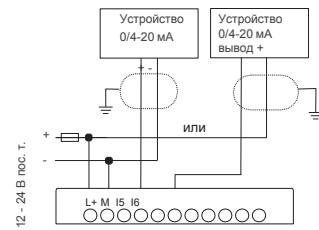
[аналоговые входы пос. т. 0-20 мА - питание (пос. т.)]
