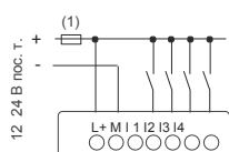
[Дискретный ввод - питание (пер. т.)]
